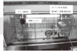
写真① 試験装置概要
